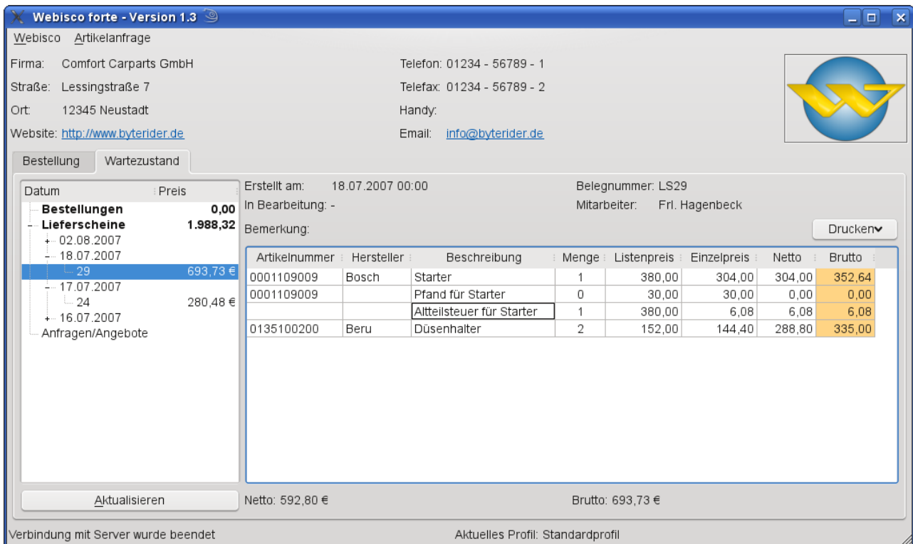
Abbildung 5: Webisco forte Hauptfenster mit aktiviertem Reiter „Bestellung“
