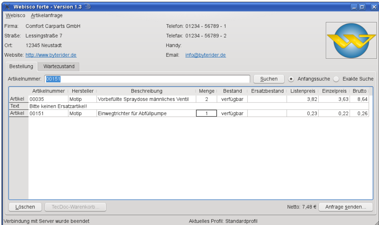
Abbildung 3: Webisco forte Hauptfenster mit aktiviertem Reiter „Bestellung“
